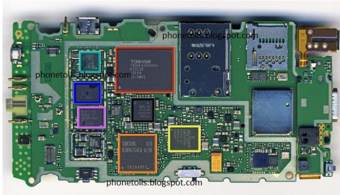
PCB Mòbil Nokia
